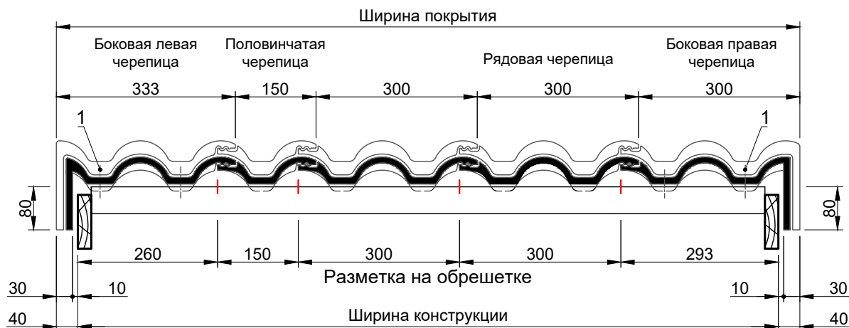
Схема укладки черепицы с применением боковой универсальной черепицы по ширине ската
